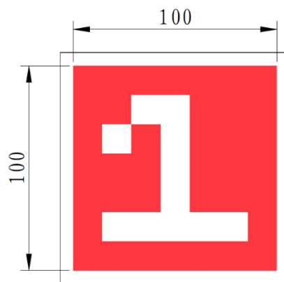
图 2-12 视觉标签有效尺寸示意图
