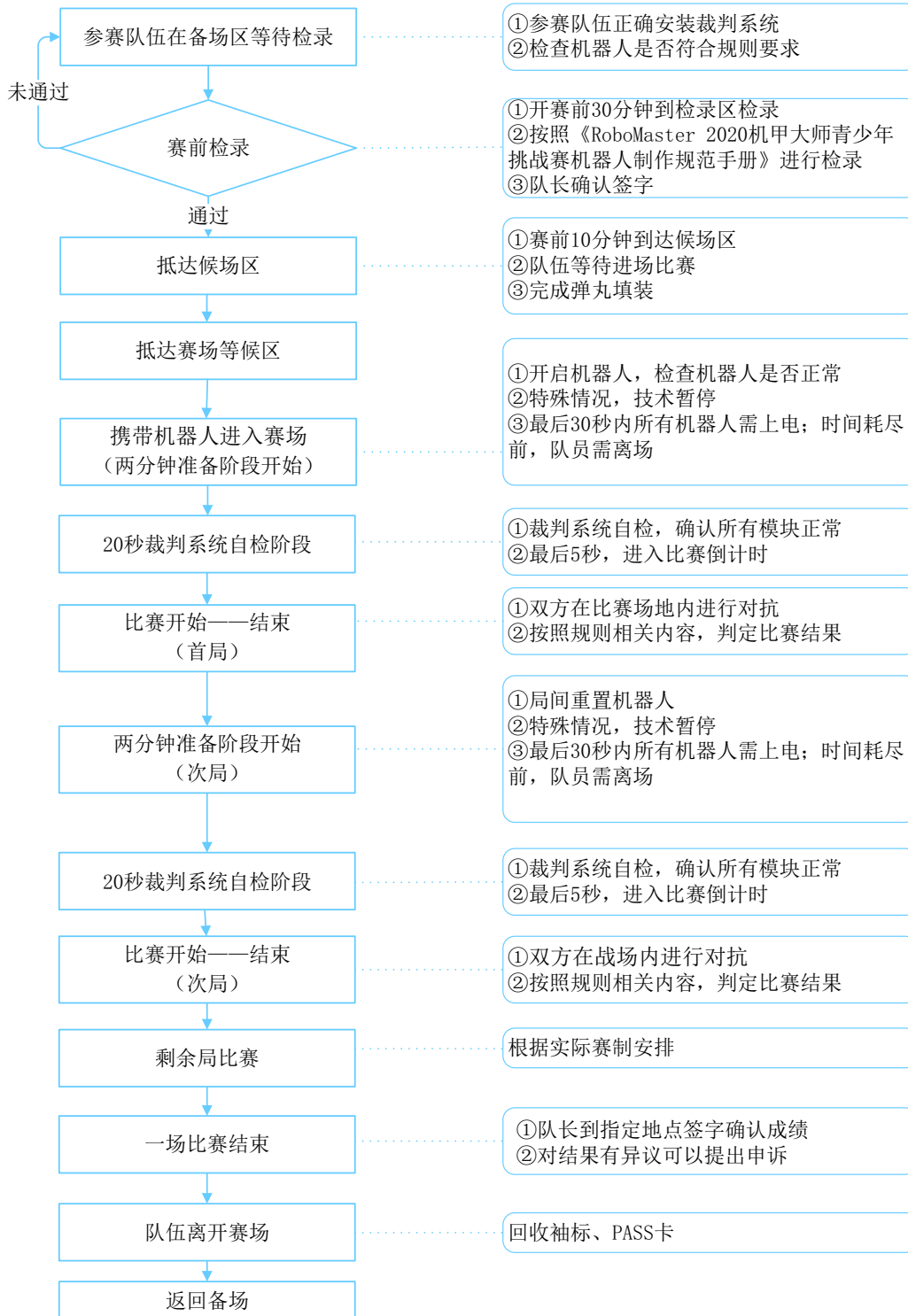
图 4-1 单场比赛流程图
