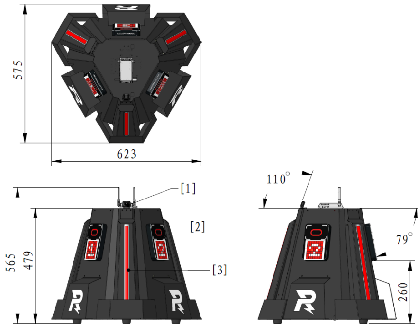
[1] 相机模块 [2] 装甲模块 [3] 基地血量灯条
