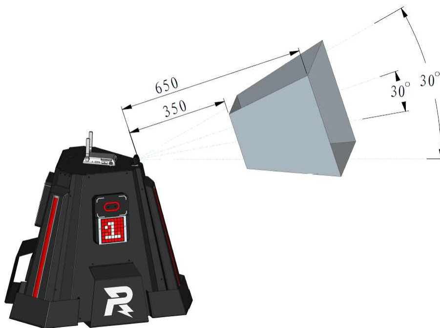
图 3-8 基地识别区示意图
