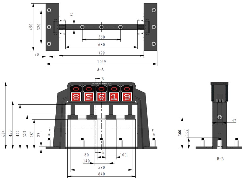
图 2-18 资源岛尺寸图
